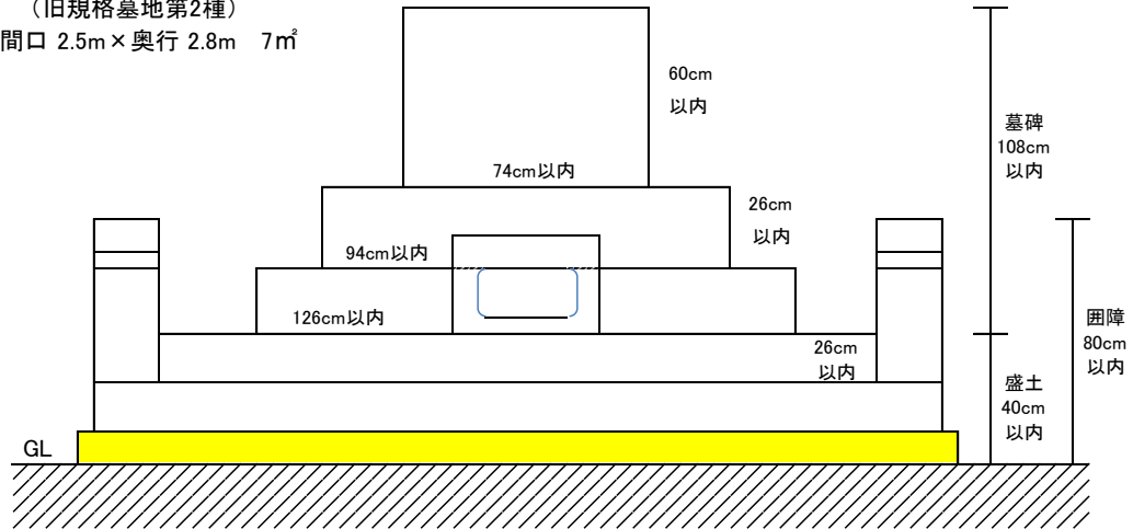
正面図
