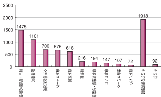
平成18年における電気火災の出火原因内訳
