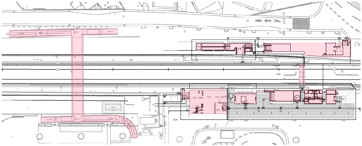
1階平面図 1 : 600
