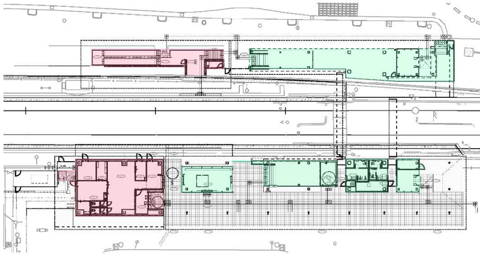
1階平面図 1:400
