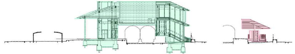
北側立面図 1:400
