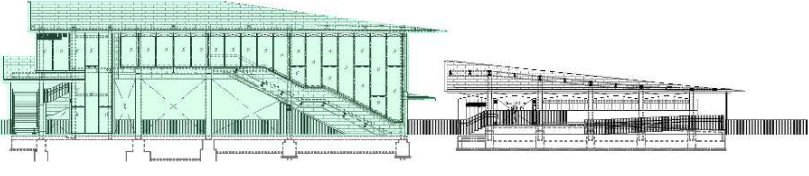
西側立面図 1 : 400
