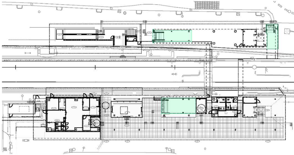
1階平面図 1 : 400
