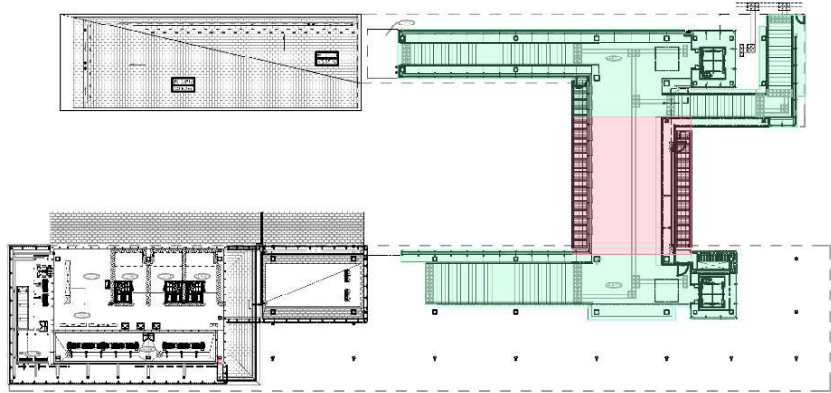
2階平面図 1 : 400
