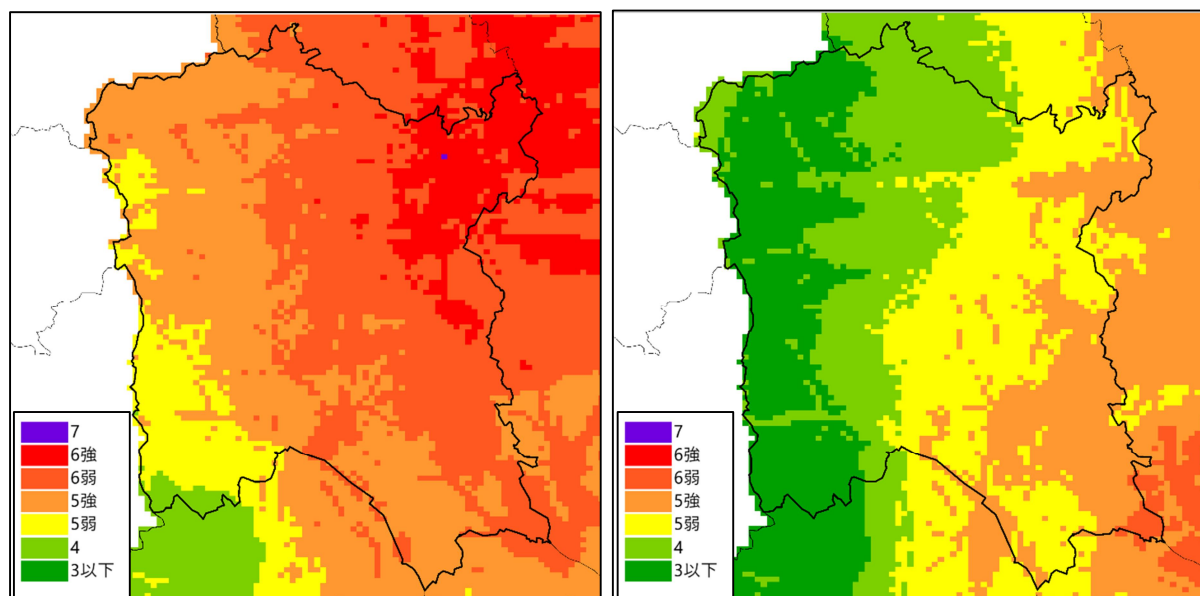
図 4 震度分布図
