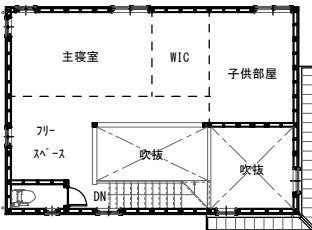
2 階平面図 (1)
