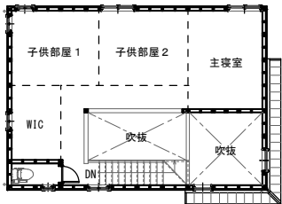
2 階平面図 (2)
