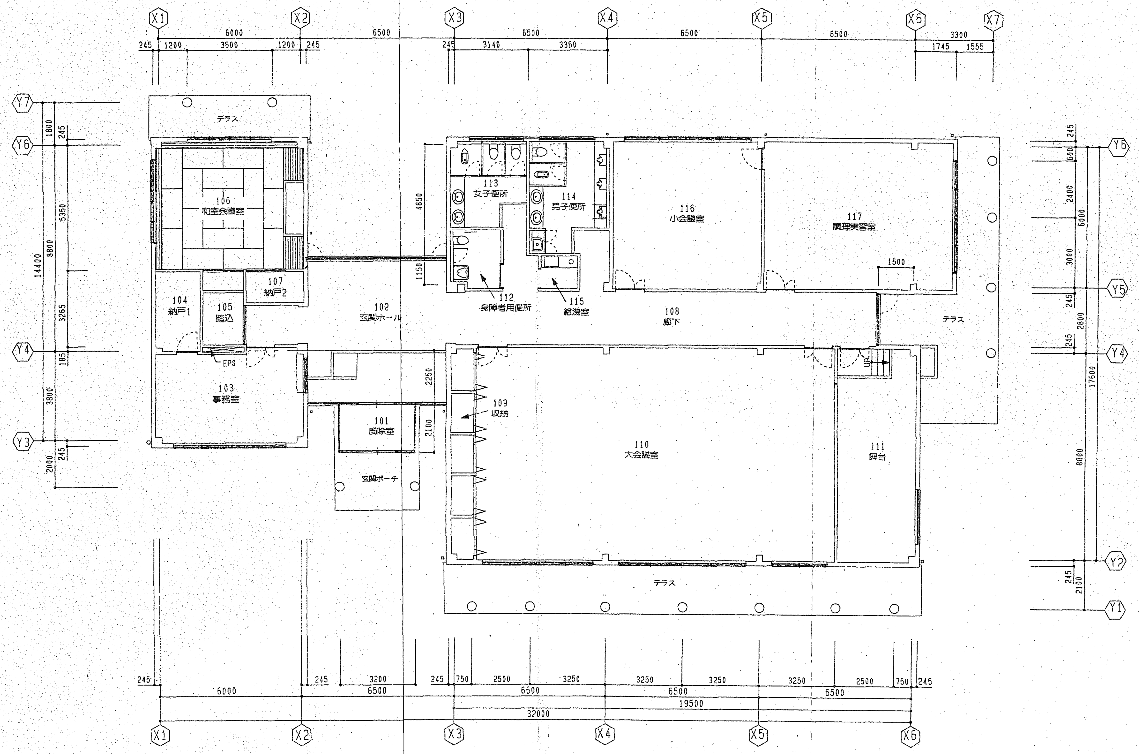
1階平面図
